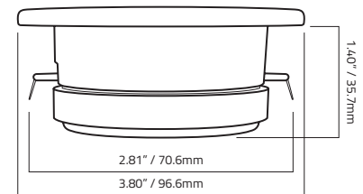
HT3PRO - TWEETER
