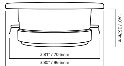
HT3PRO - TWEETER
